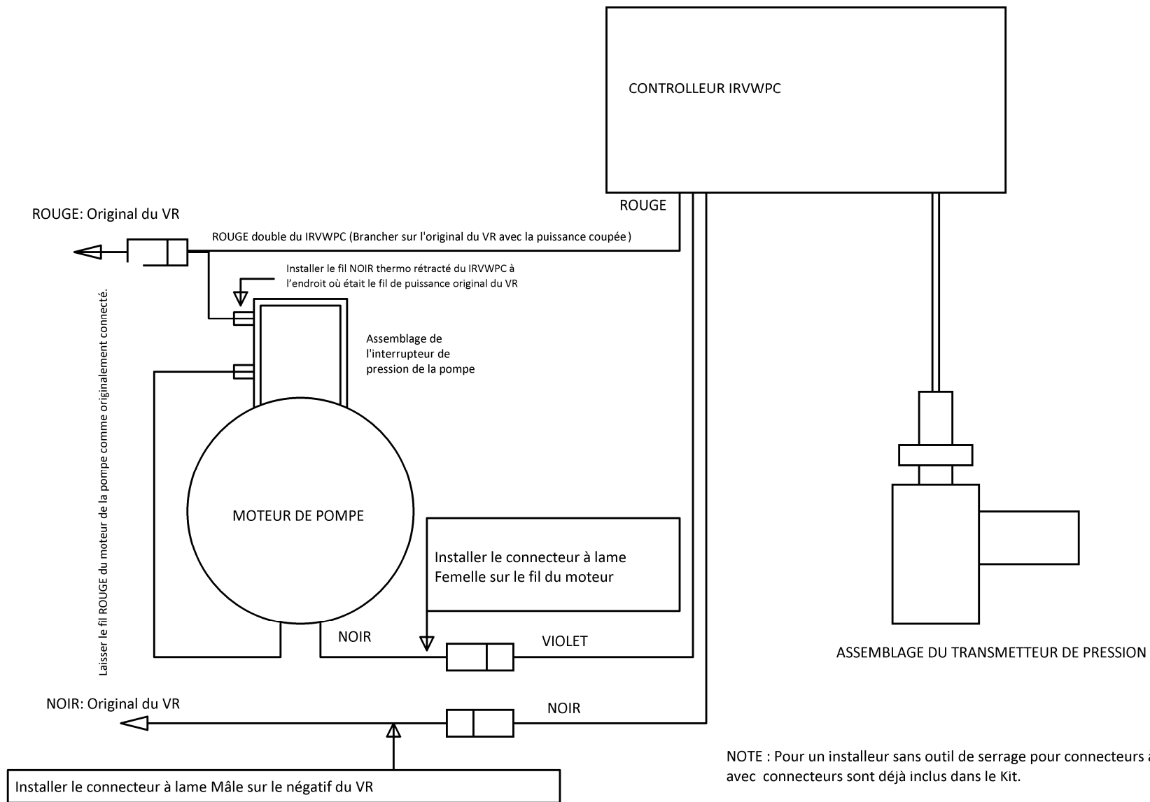
FIGURE 1: DESSIN SCHÉMATIQUE
